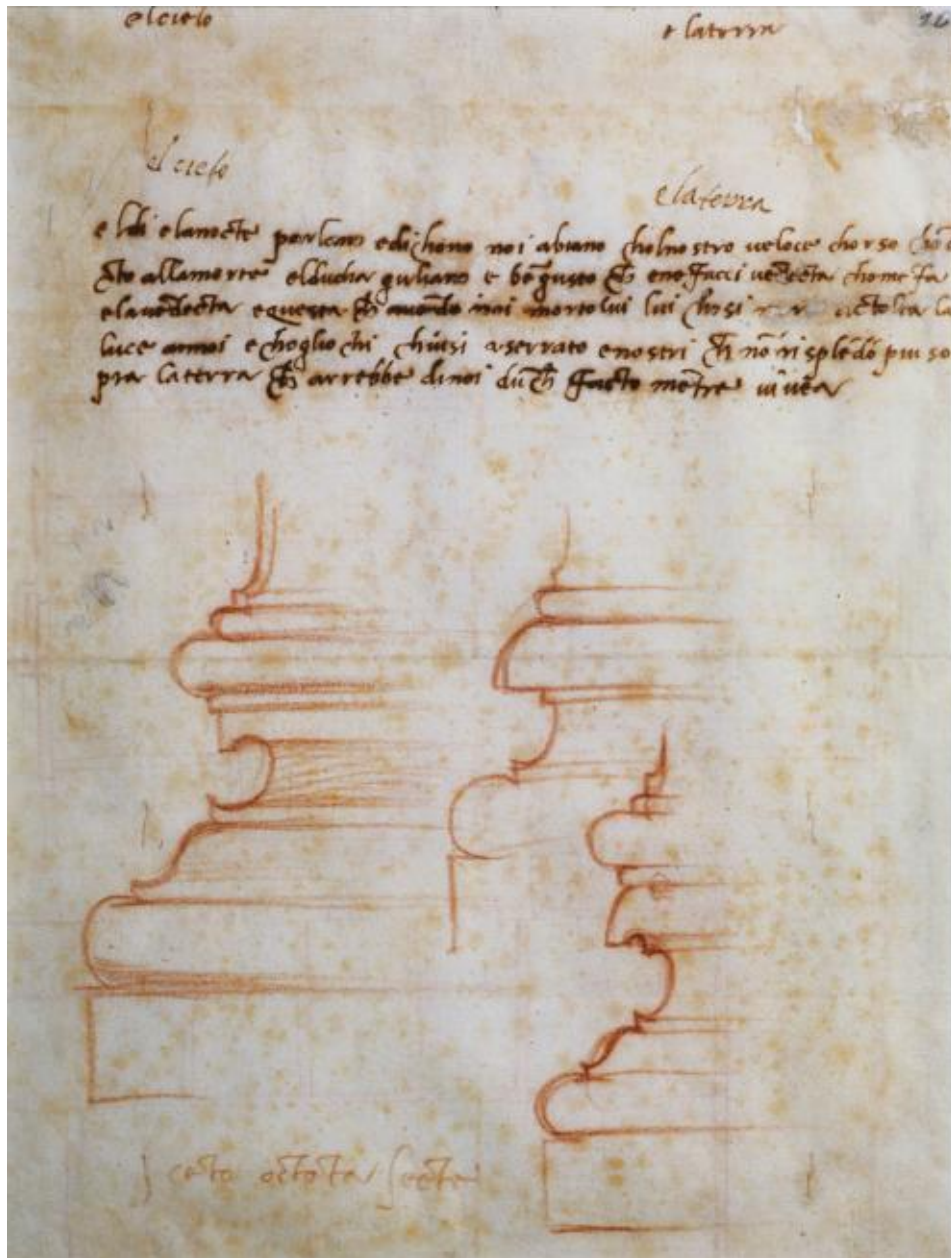
12. Michelangelo, Basi di pilastro per la Sagrestia Nuova con scritte autografe , 1524. Firenze, Casa Buonarroti, inv. 10 A
